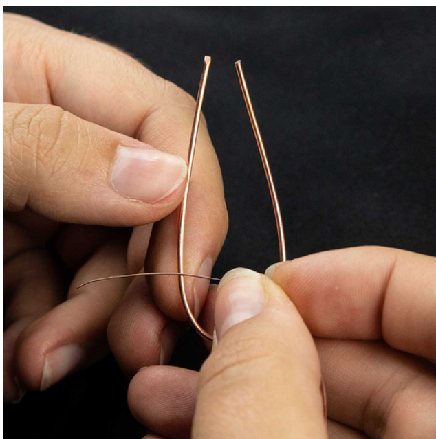
7. Vezměte si tenký drátek, nechte si cca 1 cm konec a začněte jím obtáčet tlustý drát v nejširším místě základního tvaru.
