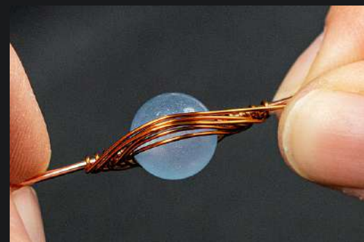
10. Na stranách se vám bude drátek hromadit, viz foto. Nehromadte jednotlivé otáčky na sebe, ale hezky pod sebe.
